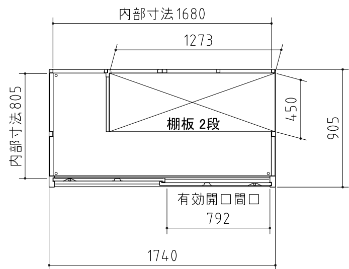
平面図
